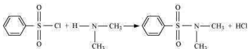
Benzenesulphonyl chloride
