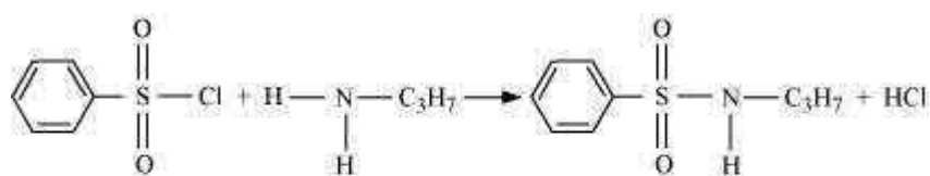
Benzenesulphonyl chloride
